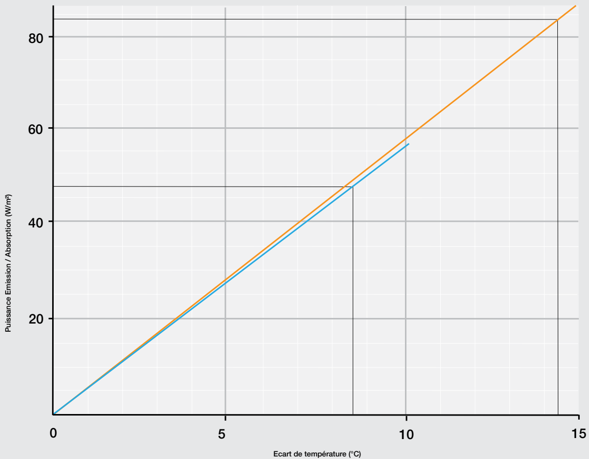
CD-4 - Performance en chauffage et rafraîchissement (Parement : plaque de plâtre 0.04m 2 .K/W)
