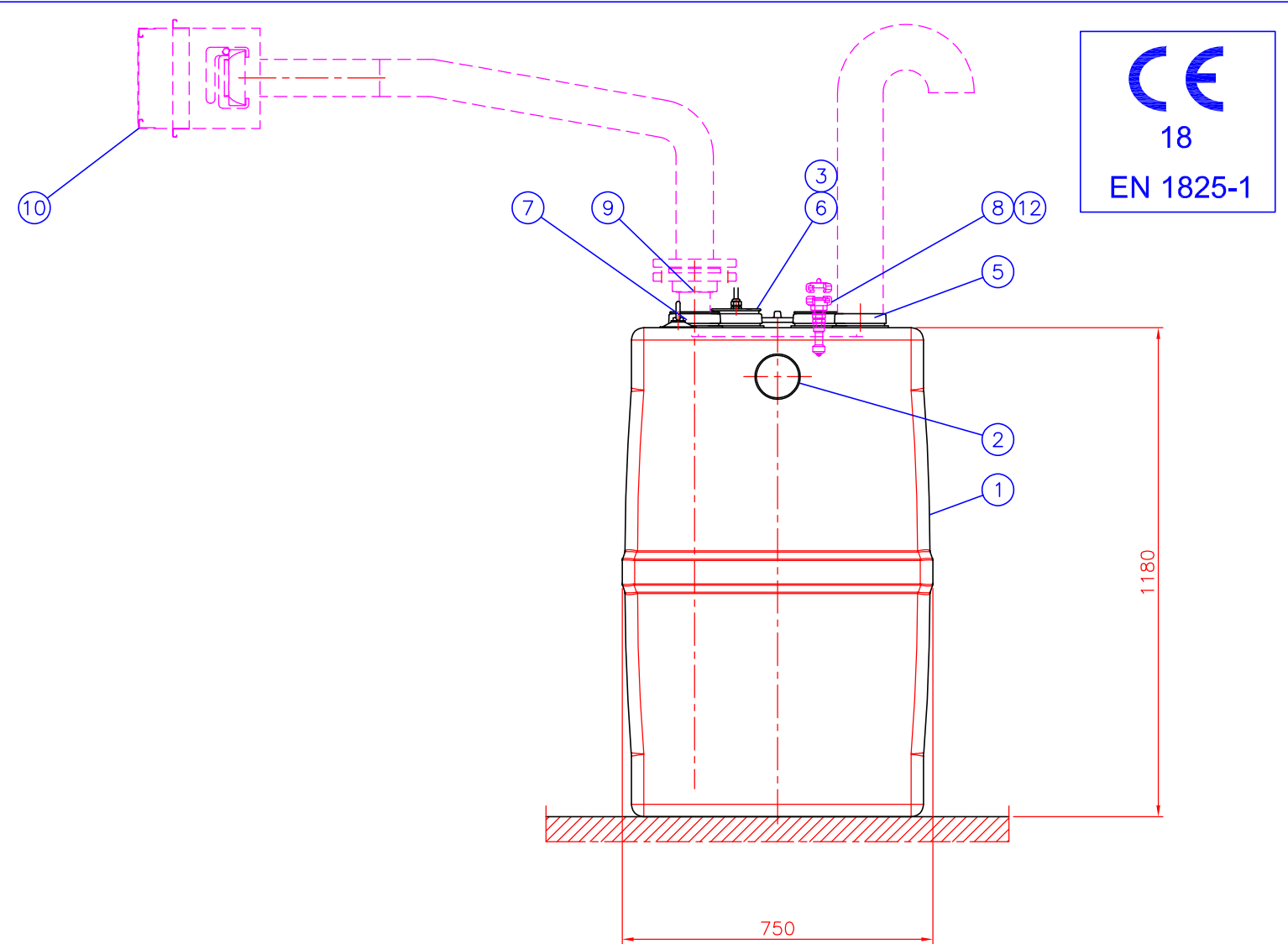
Rasvanerottimen asennus sisätilaan, lattian päälle.
