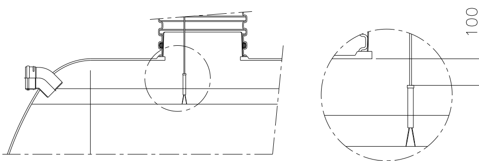
Kuva 12. Anturin asennus LOKA 15000 – 80000
