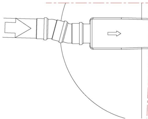
Kuva 10. "Joustava" tuloyhde kahdella 15° kulmayhteellä.
