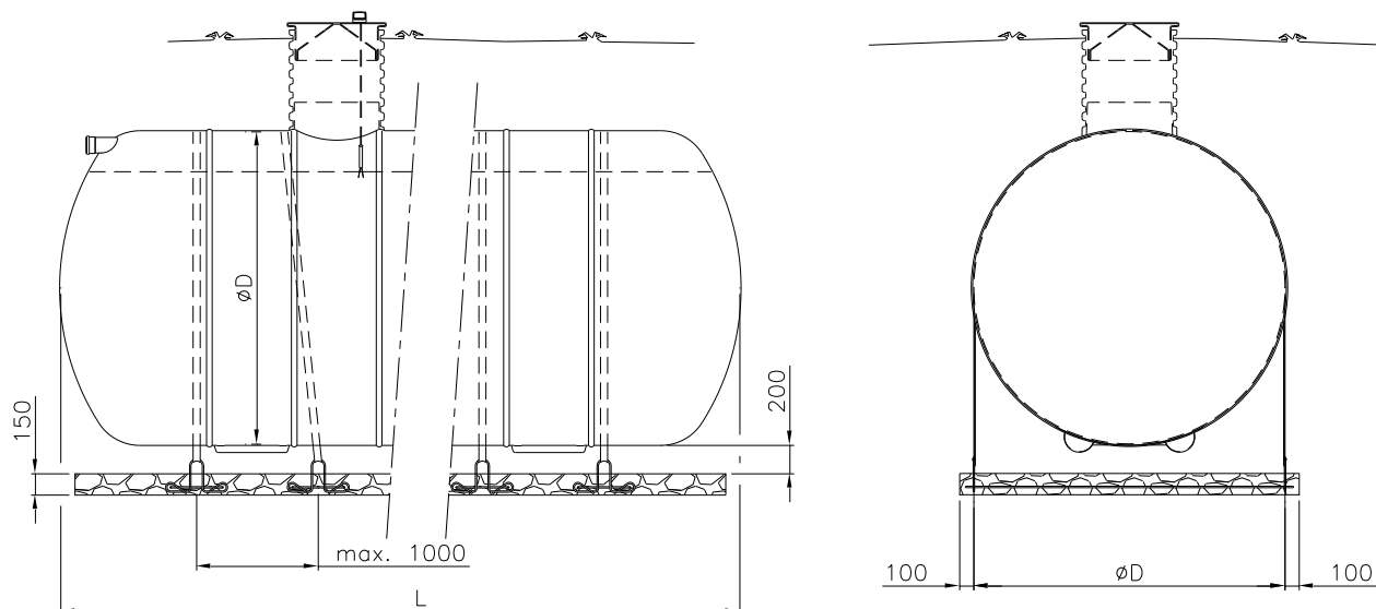
Kuva 7. LOKA 15000 - 80000 ankkurointi betonilaattaan.
