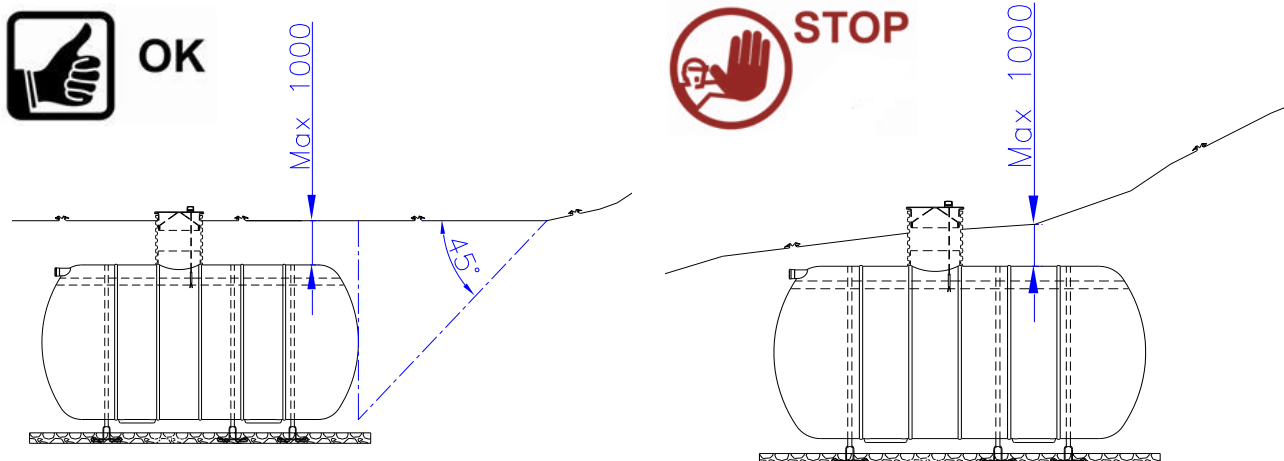
Kuva 8. Lokasäiliöiden rinneasennus.
