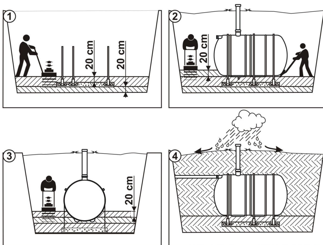
Kuva 9. Kaivannon täyttäminen.
