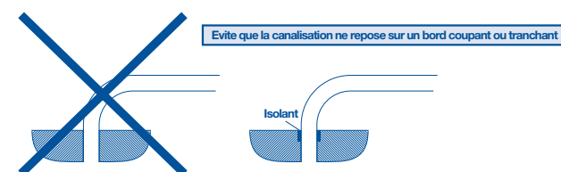
Figure 6 Protection des conduites Wavin Tigris émergeant d'un plancher ou d'une paroi
