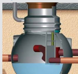
Регулирующие колодцы Labko FRW
