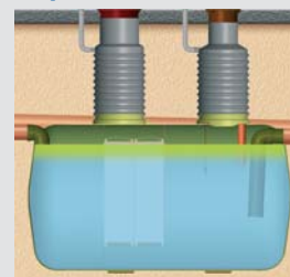
Нефтемаслоотделители EuroPEK Roo
