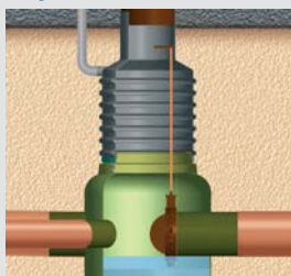
Колодцы для отбора проб с запорным вентилем EuroNOK FRW и EuroNOK
