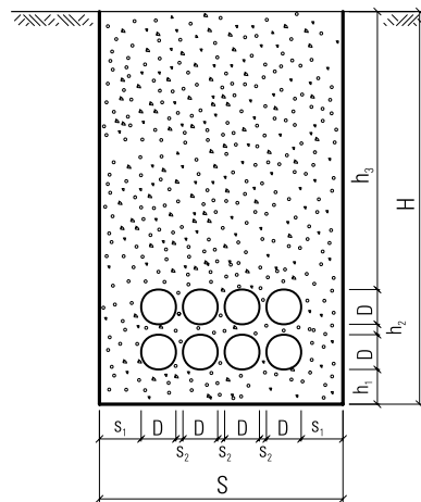
Fig. 4: Lægning af flere rør i en kabelrende
