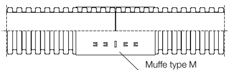
Fig. 8: Samling af rør med sandtæt muffe, type M
